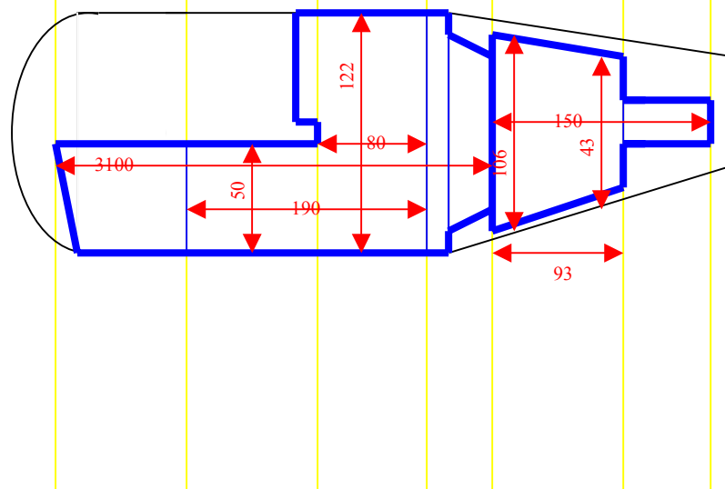
Vue de dessus de l'hélicoptère
